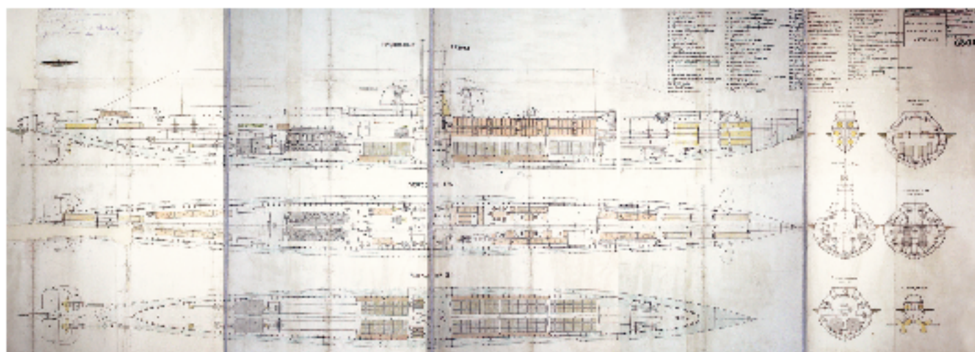
Практичный чертёж общего расположения подводной лодки типа «Декабрист»
